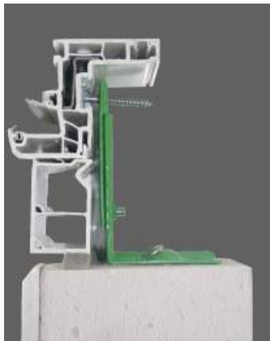
Montage sur dormant PVC
